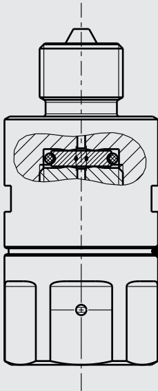
Cross-section DIPS / Querschnitt DIPS
