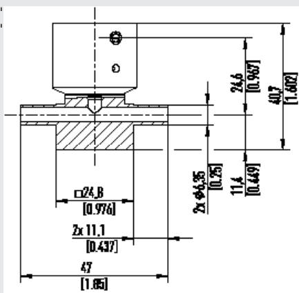
Raccord à souder 1/4" Raccord à souder 1/4"
