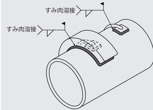
図1:溶接モード図
