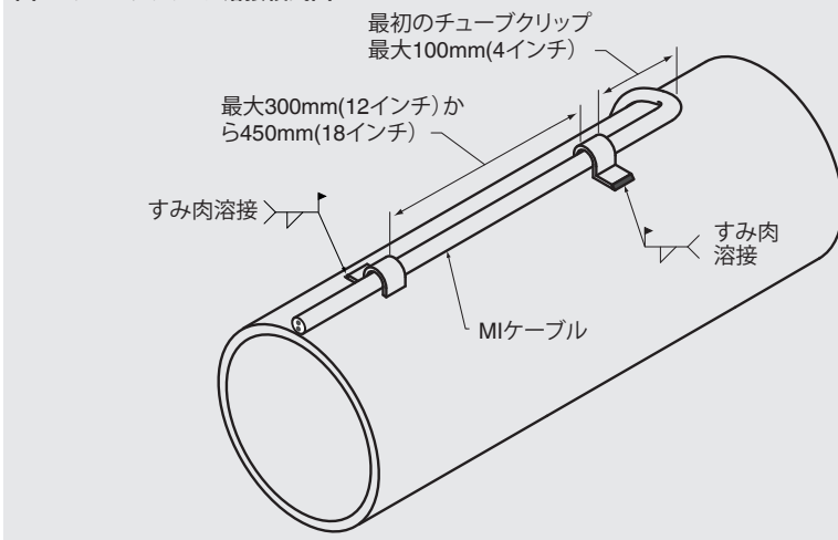
図2:チューブクリップ溶接モード図
