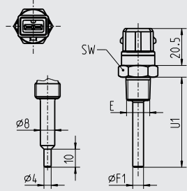
Bajonett-Stecker, DIN 72585
